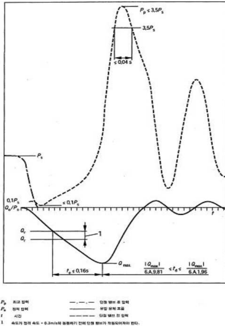
그림 3 유압 유체유량, 램쳐 밸브의 전단 및 후단의 압력
