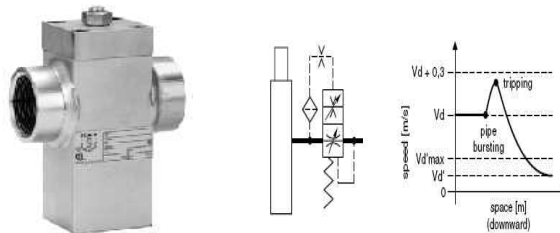
그림 1 립쳐 밸브
