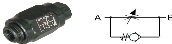
그림 2 단방향 유량제한기
